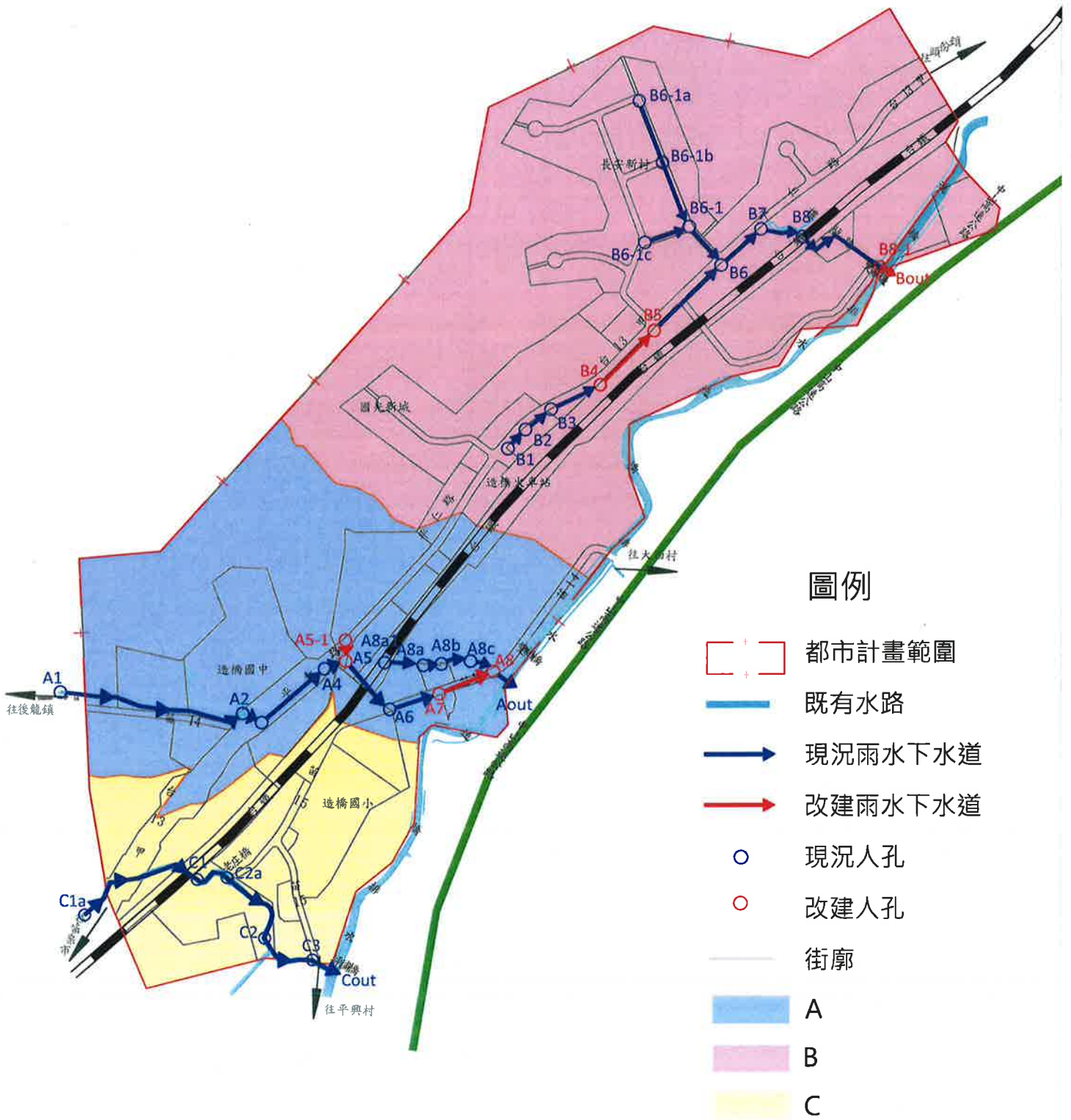
造橋鄉雨水下水道排水區域範圍圖
