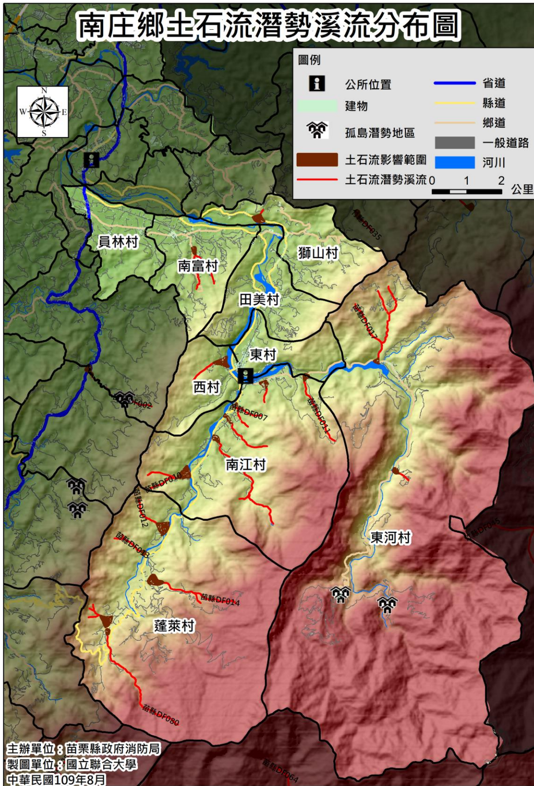
圖 1.5 南庄鄉土石流災害潛勢圖
