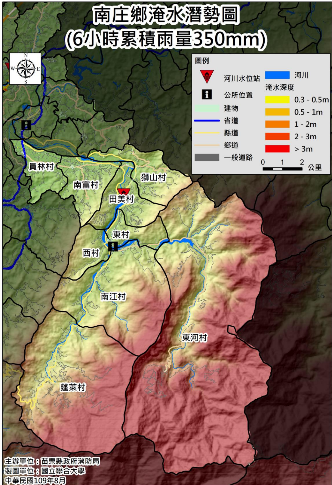
圖 1.1 南庄鄉 6 小時淹水潛勢圖
