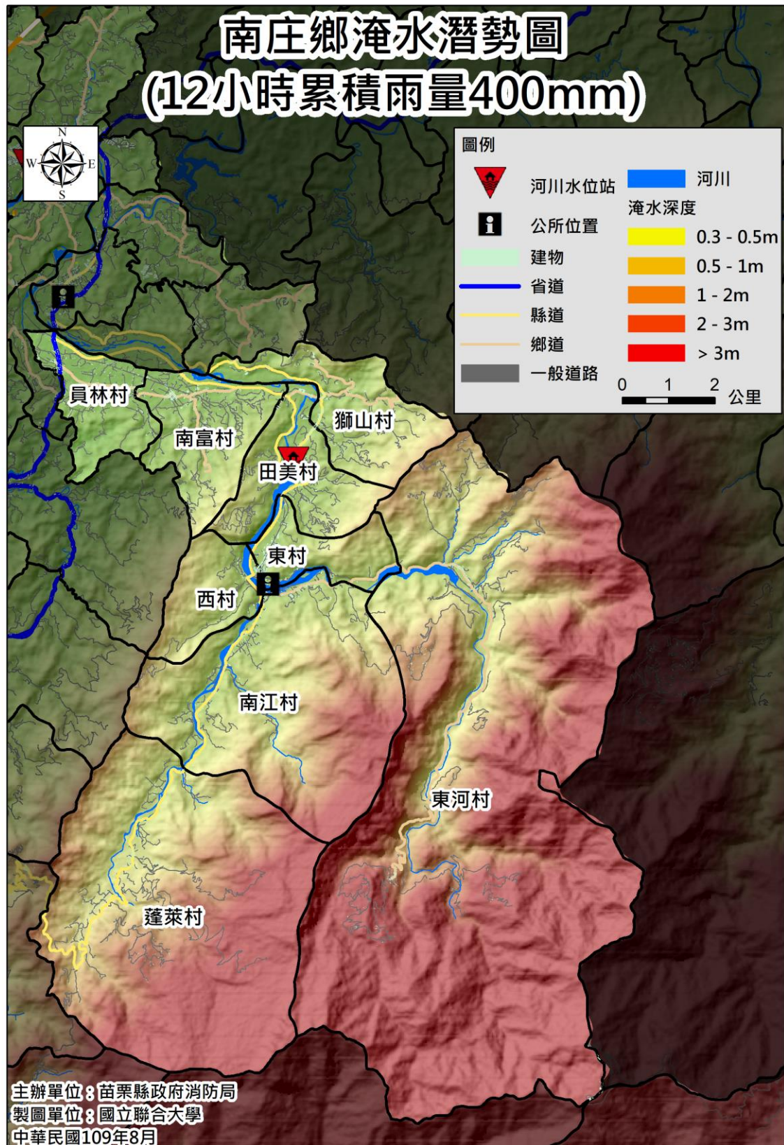
圖 1.2 南庄鄉 12 小時淹水潛勢圖
